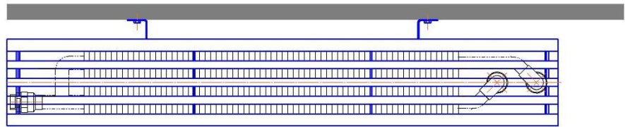
Монтажная схема настенного конвектора "Элегант 110х400-2то Стен" с нижним подключением (присоединительная резьба - 1/2")
