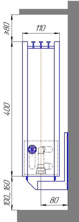
Монтажная схема настенного конвектора "Элегант 110х400-2то Стен" с нижним подключением (присоединительная резьба - 1/2")
