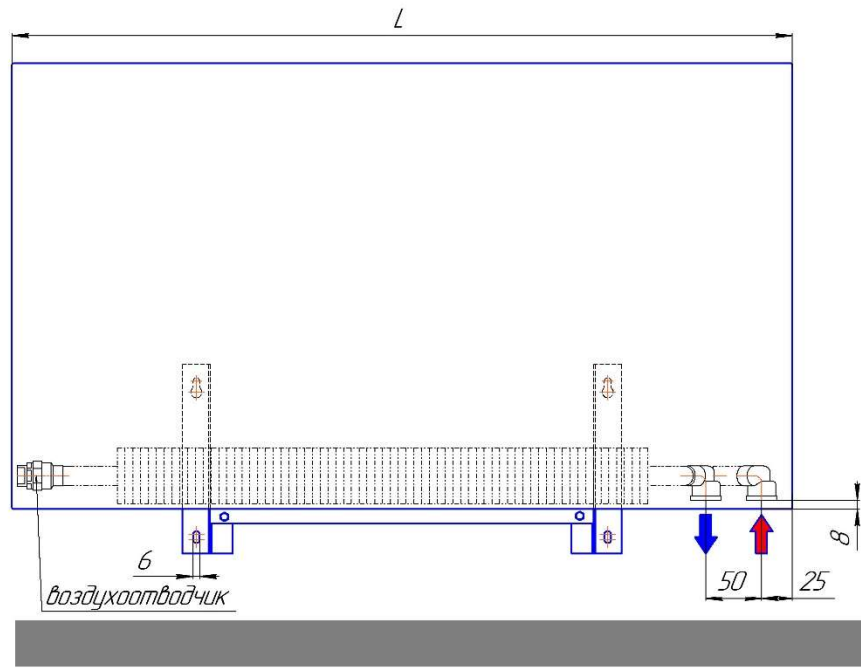
Монтажная схема настенного конвектора "Элегант 110х400-1то Стен" с нижним подключением (присоединительная резьба - 1/2")
