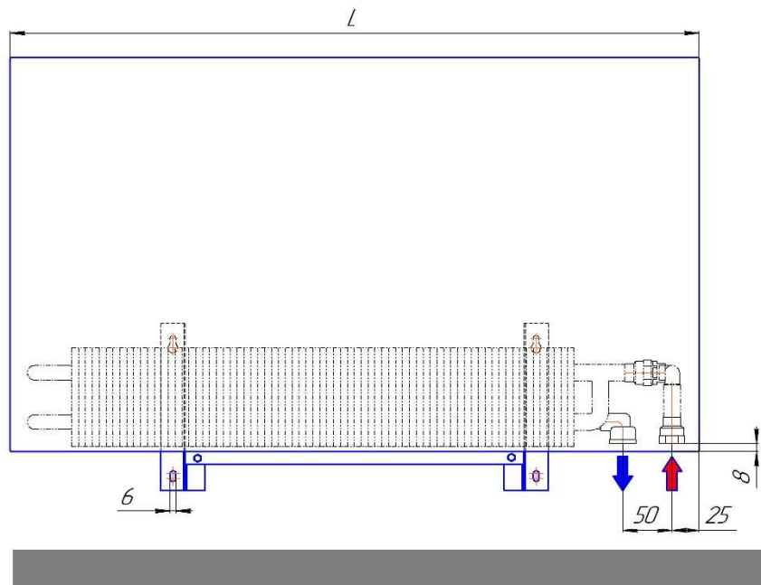
Монтажная схема настенного конвектора "Элегант 110х400-2то Стен" с нижним подключением (присоединительная резьба - 1/2")
