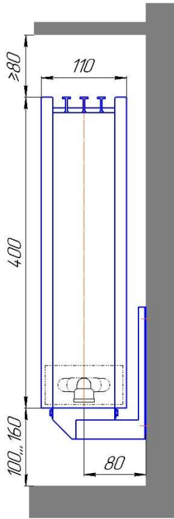
Монтажная схема настенного конвектора "Элегант 110х400-1то Стен" с нижним подключением (присоединительная резьба - 1/2")
