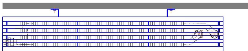
Монтажная схема настенного конвектора "Элегант 110x250-2то Стен" с нижним подключением (присоединительная резьба - 1/2")
